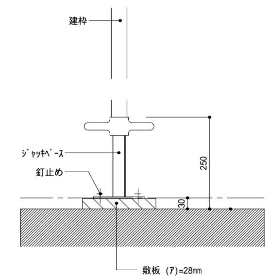
支保工脚部詳細図 S=1/10
