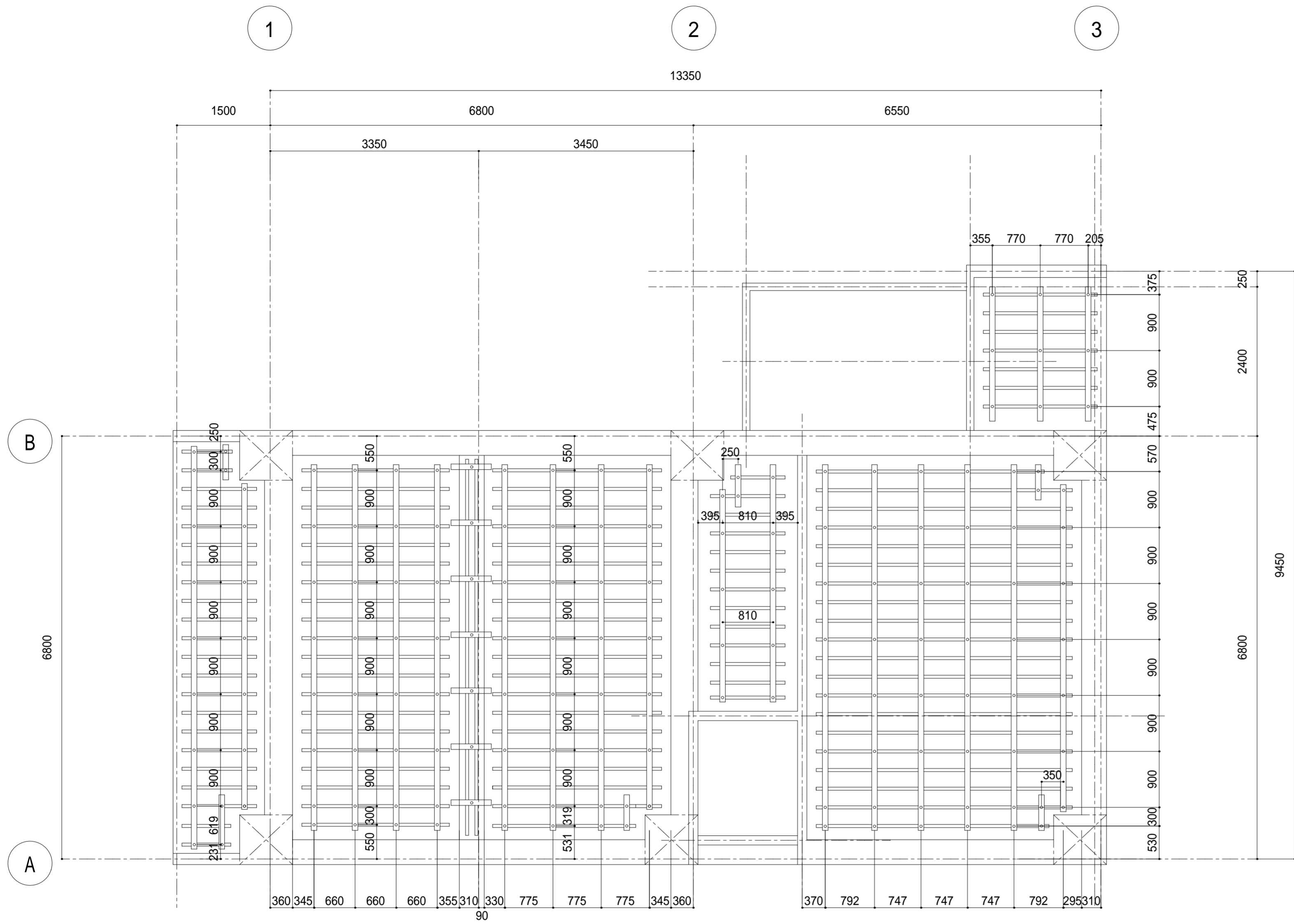
型枠支保工図 (1/50)
